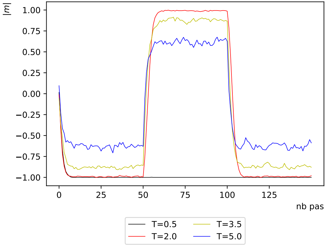
Aimantation en présence d'un champ magnétique variant de h=-1.5 à +1.5 , N=32, k=50
